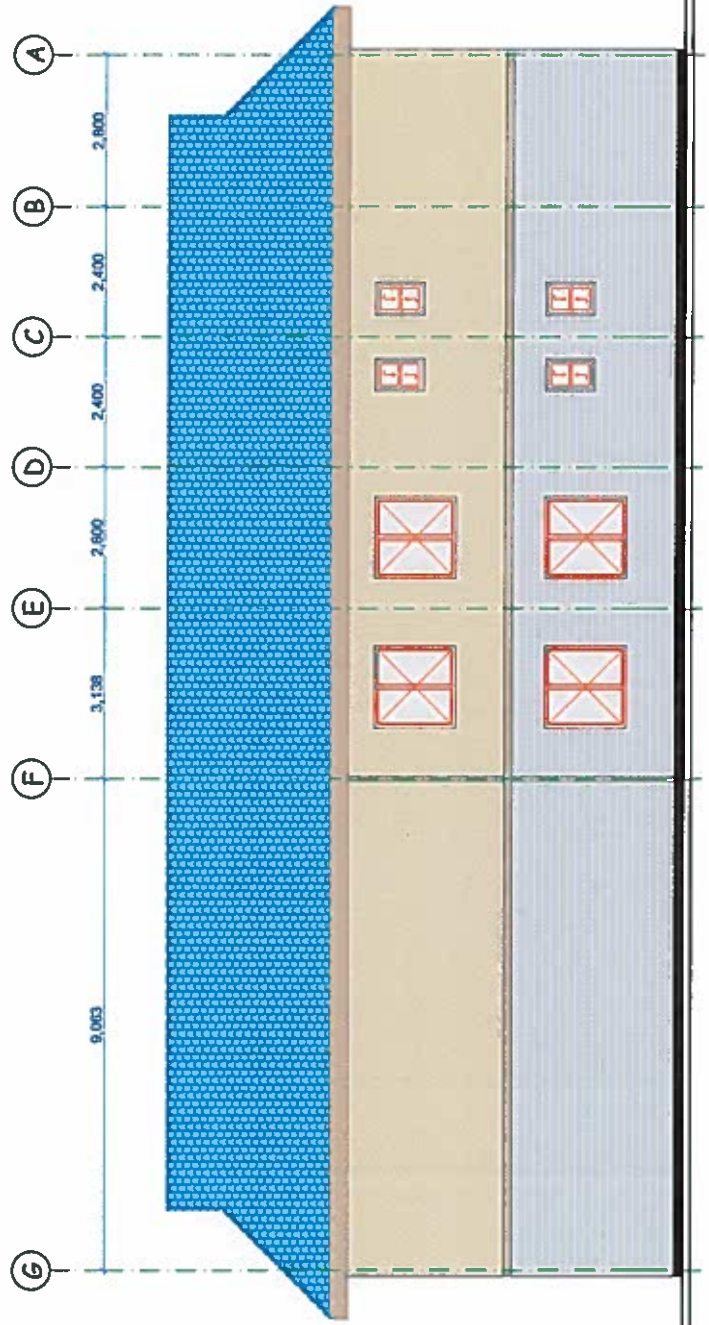
ELEVATION 02
